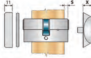
Tenax kalınlık seçenekleri (X) Barel çıkıntısına göre (S)
